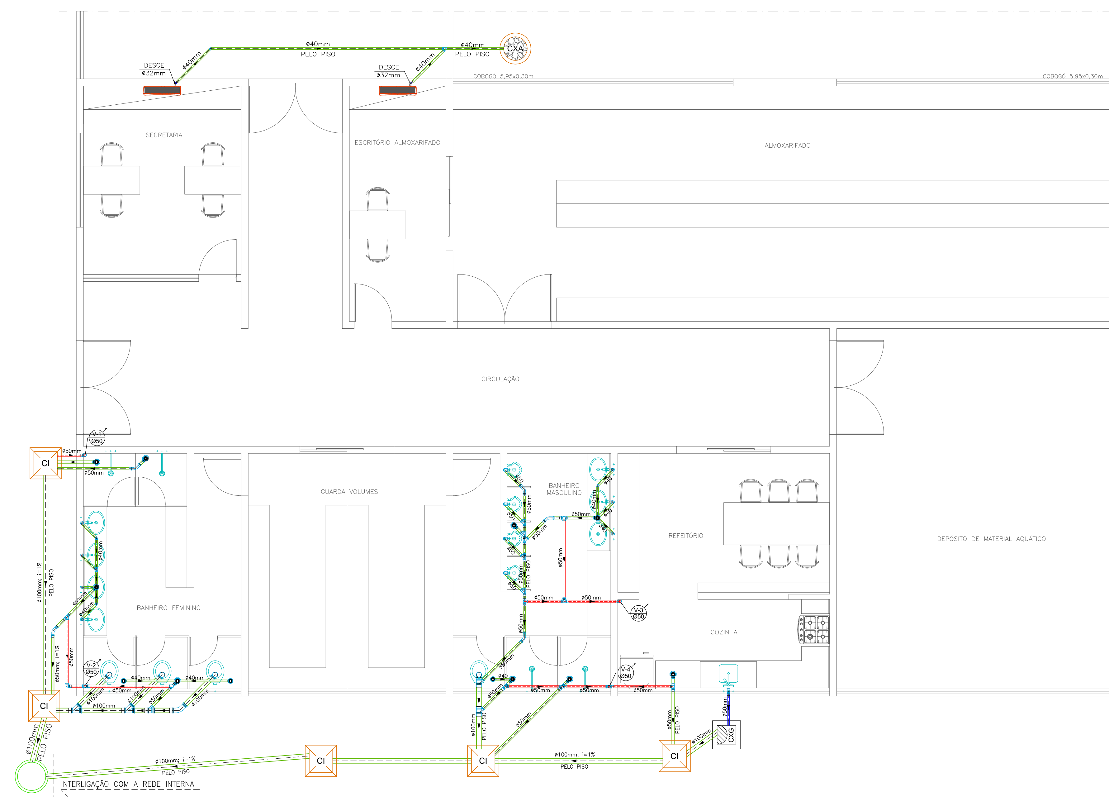
PLANTA BAIXA - BLOCO 14 ESCALA: 1/50
