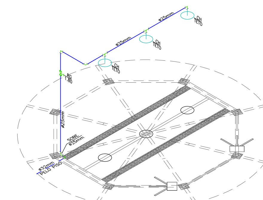
ISOM - PEDILUVIO (BLOCO 05) ESCALA: 1/50
