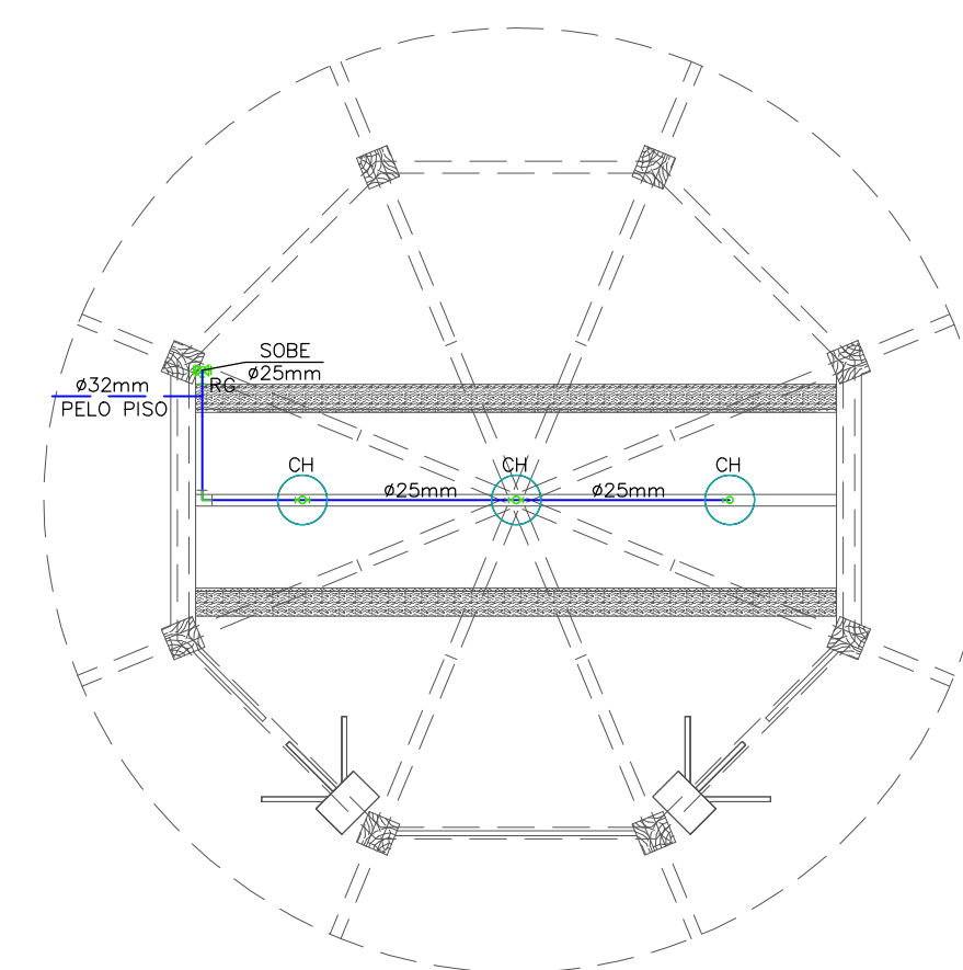
PLANTA BAIXA - BLOCO 05 ESCALA: 1/50
