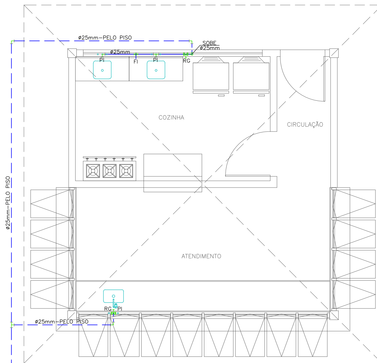
PLANTA BAIXA - BLOCO 09 ESCALA: 1/50
