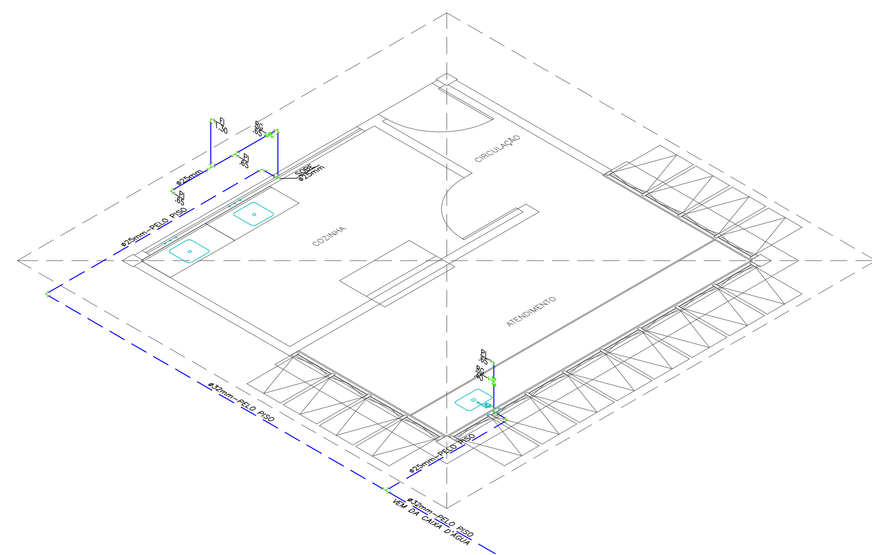
ISOM - LANCHONETE (BLOCO 09) ESCALA: 1/50
