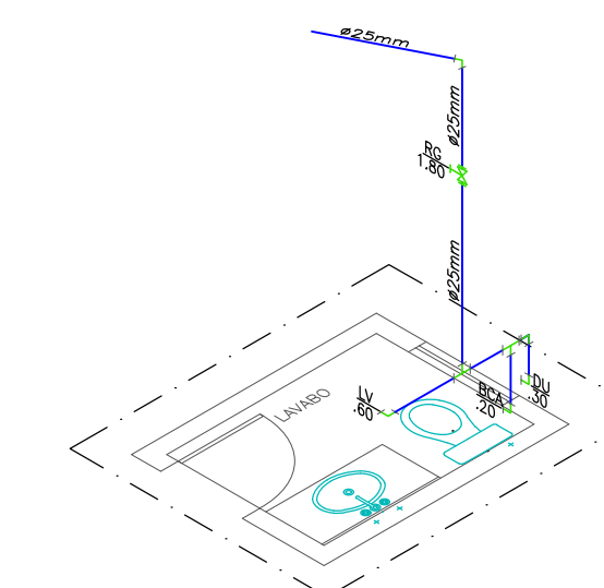
ISOM - LAVABO (BLOCO 15) GERRÊNCIA ESCALA: 1/50
