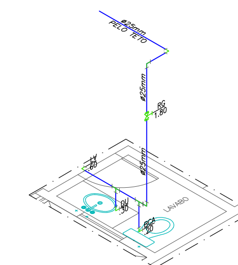
ISOM - LAVABO (BLOCO 15) BILHETERIA ESCALA: 1/50
