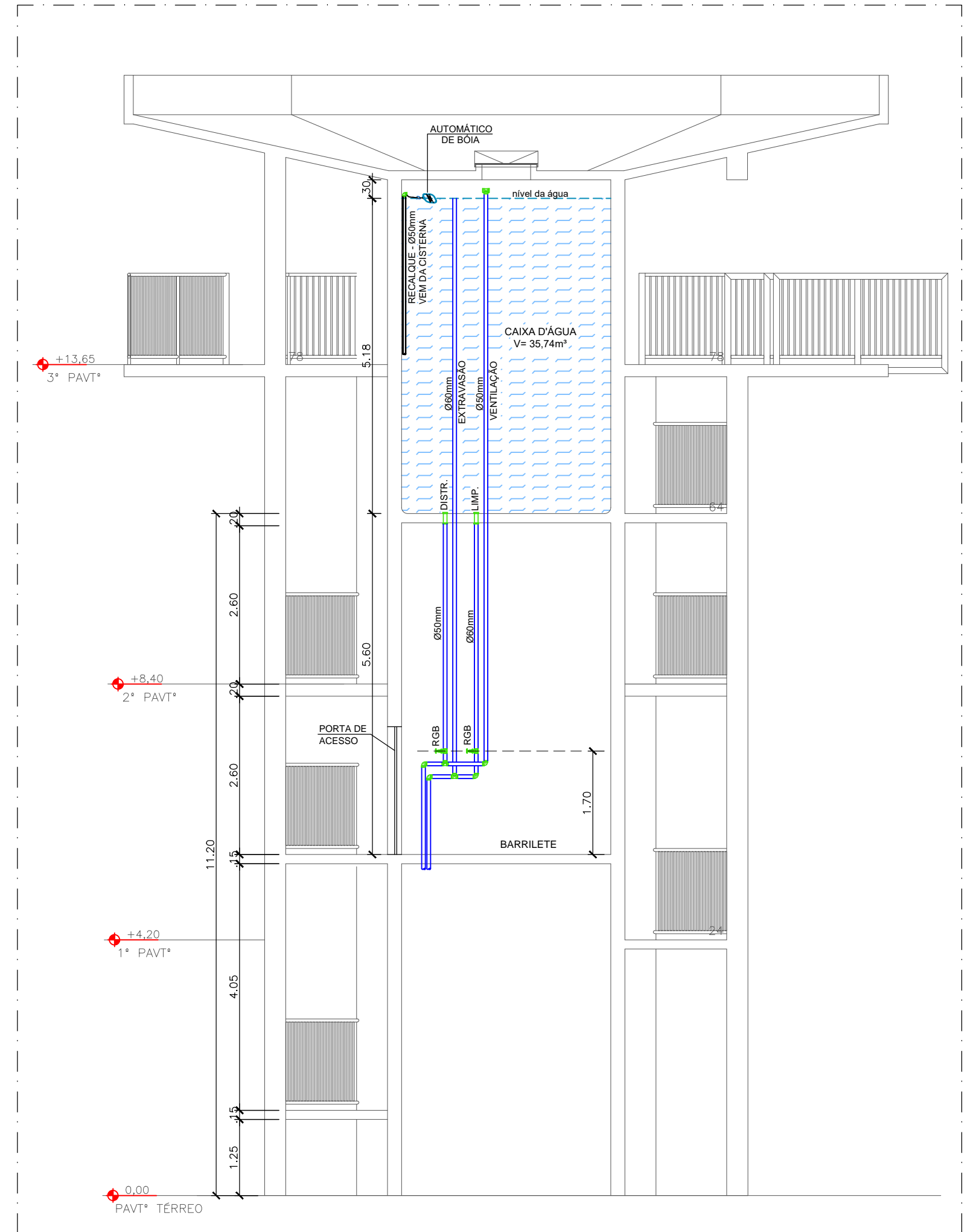
CORTES ESQUEMÁTICO - CAIXA D'ÁGUA DE CONSUMO (BLOCO 06) ESCALA: 1/75
