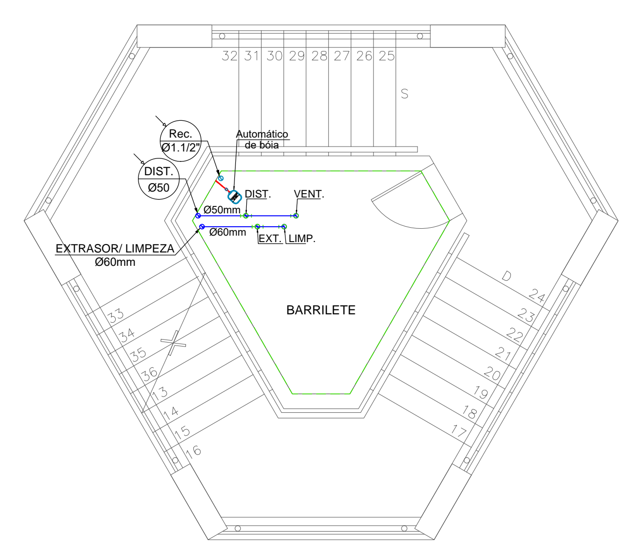
PLANTA BAIXA 1º PAVTO - BARRILETE CX. D'ÁGUA ESCALA: 1/50
