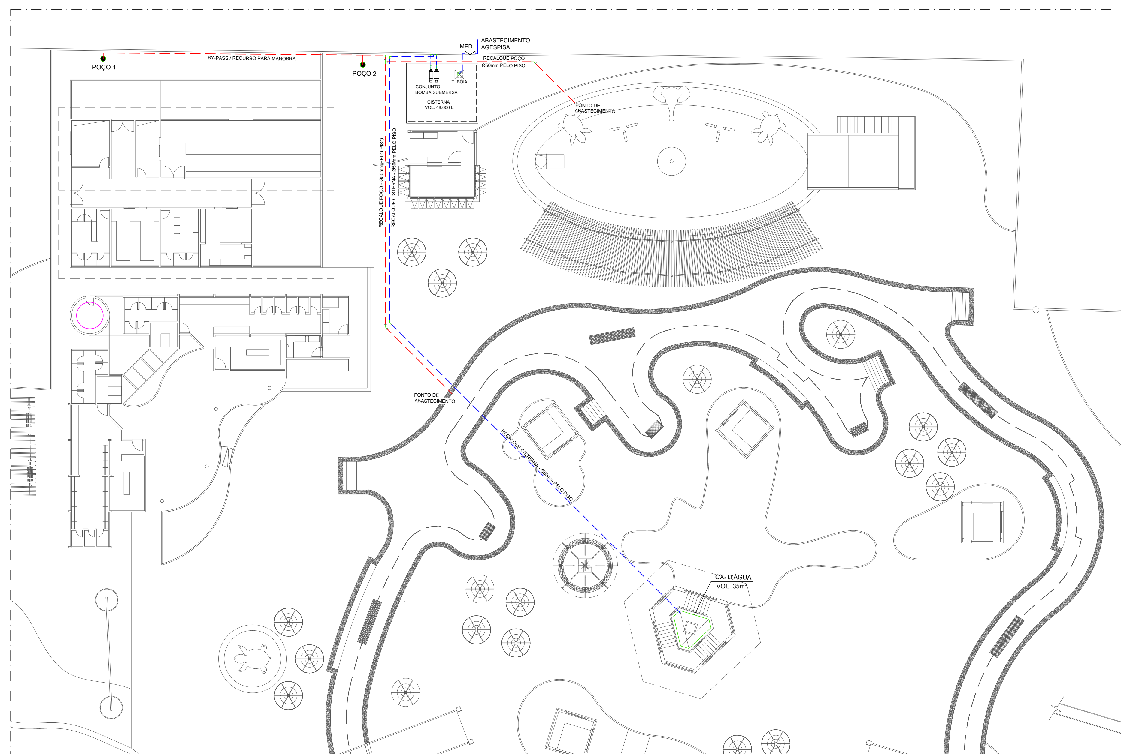
PLANTA BAIXA - ABASTECIMENTO RESERVATÓRIO AGESPISA E PISCINAS ESCALA: 1/200
