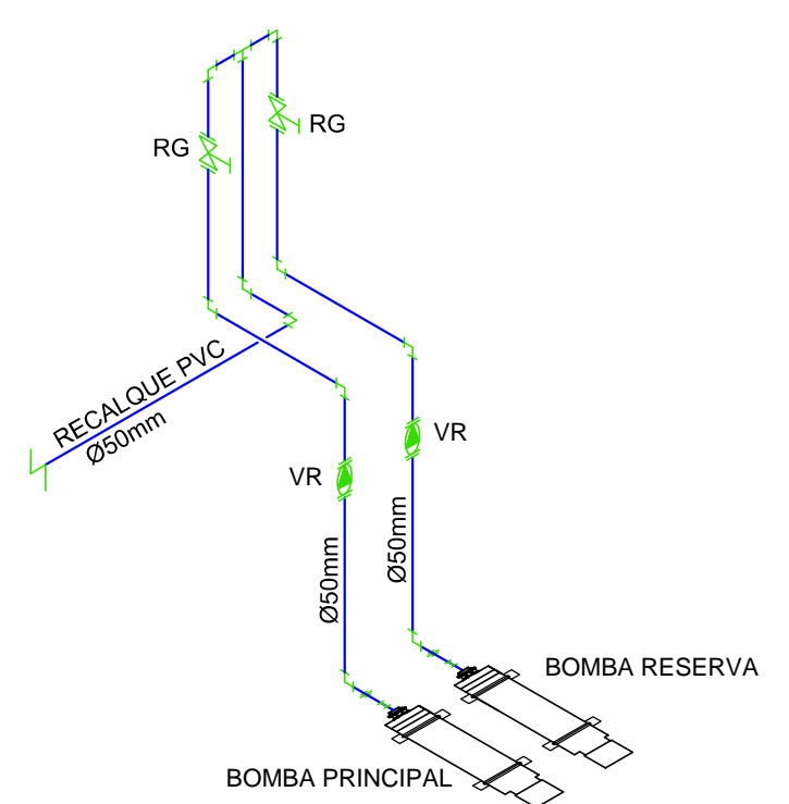
ESQUEMA ISOMÉTRICO - REGISTRO DE MANOBRAS BOMBAS DAS CISTERNAS SEM ESCALA
