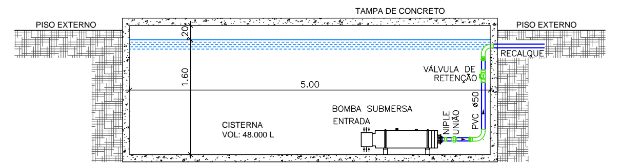
CORTE A - A (CISTERNA) SEM ESCALA
