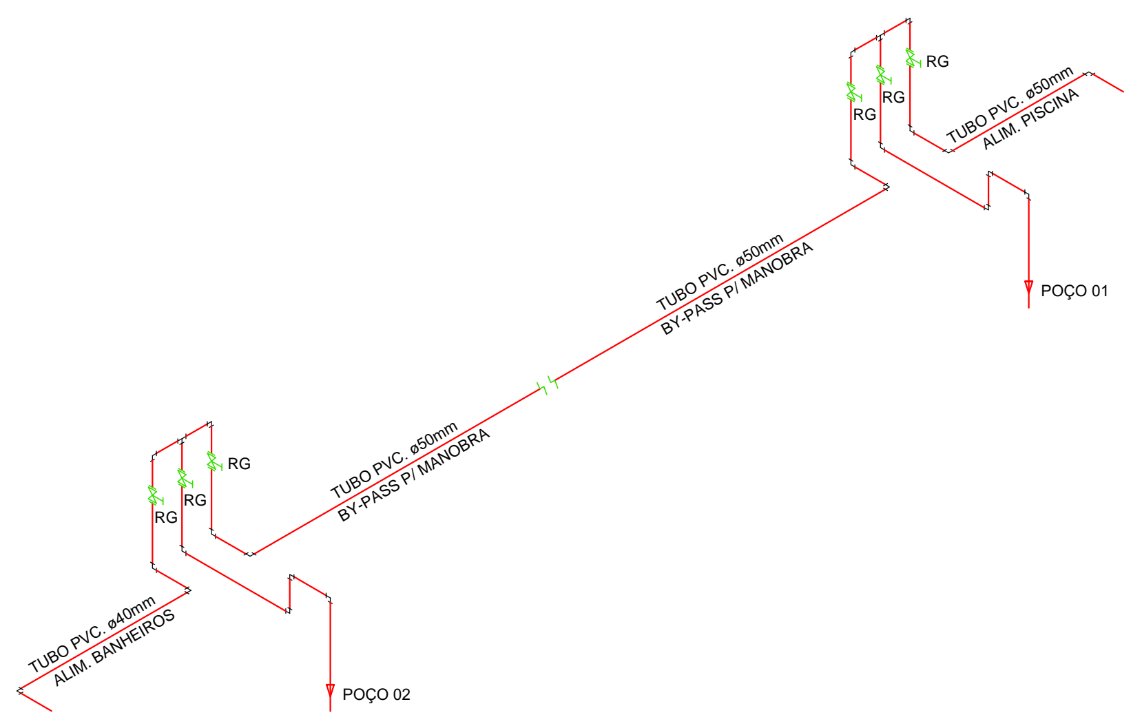
ESQUEMA ISOMÉTRICO - REGISTRO DE MANOBRAS DOS POÇOS SEM ESCALA
