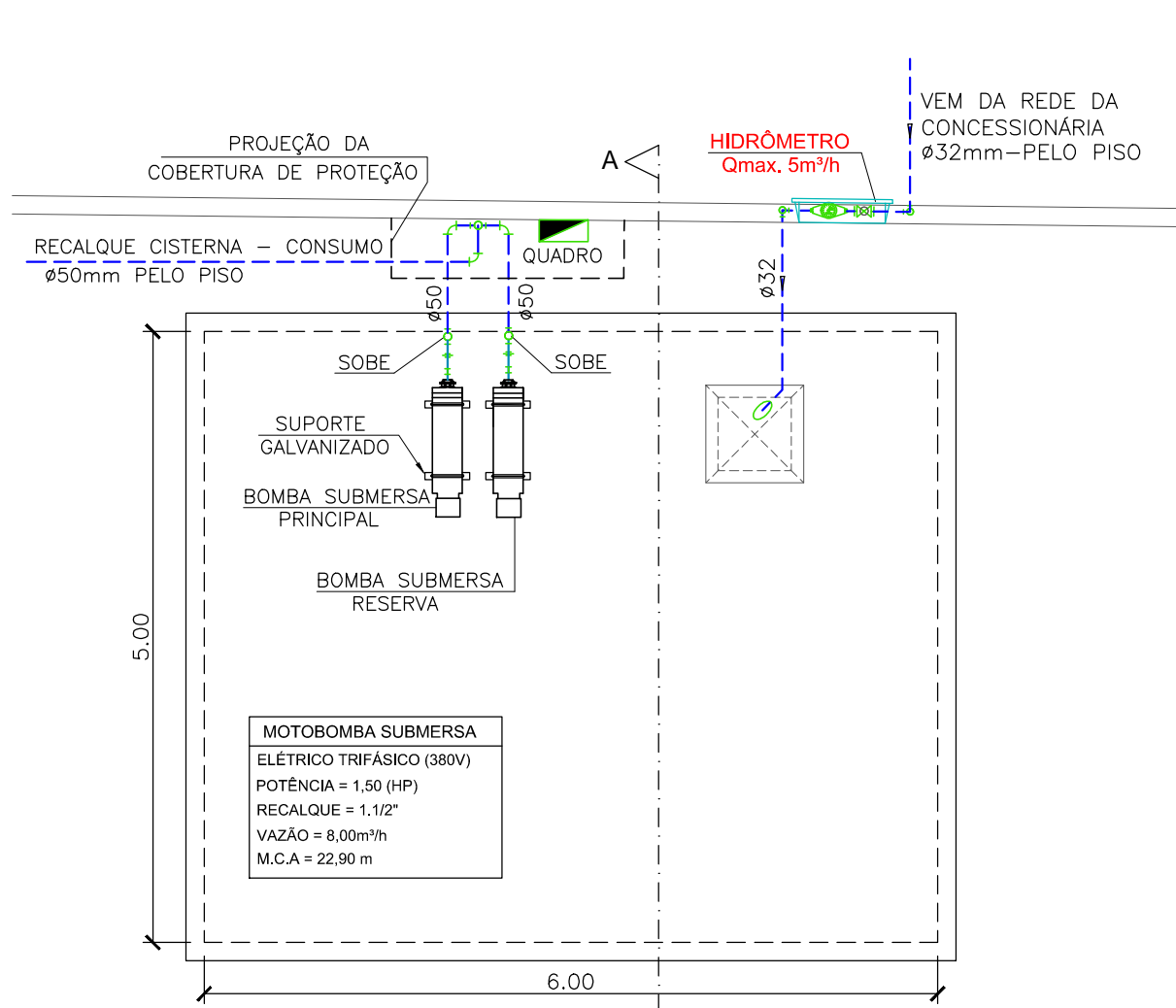
PLANTA BAIXA - CISTERNA SEM ESCALA
