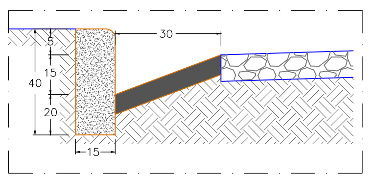
DETALHE - SARJETA SEM ESCALA (COTAS EM CM)
