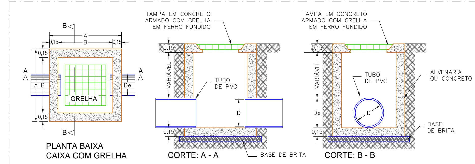
DETALHE - CAIXA PLUVIAL (CXP) COM GRELHA SEM ESCALA (COTAS EM METROS)
