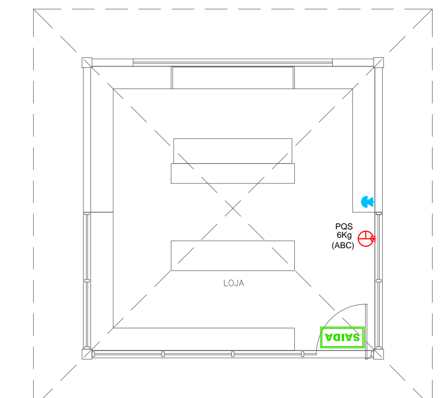
PLANTA BAIXA - BLOCO 10 (LOJA) ESCALA: 1/75
