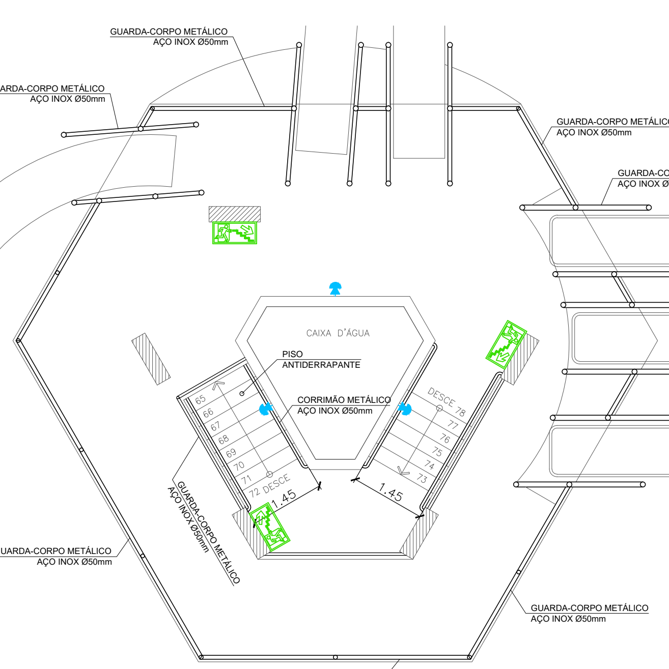
PLANTA BAIXA 3º PVTO - BLOCO 06 (TORRE) ESCALA: 1/75
