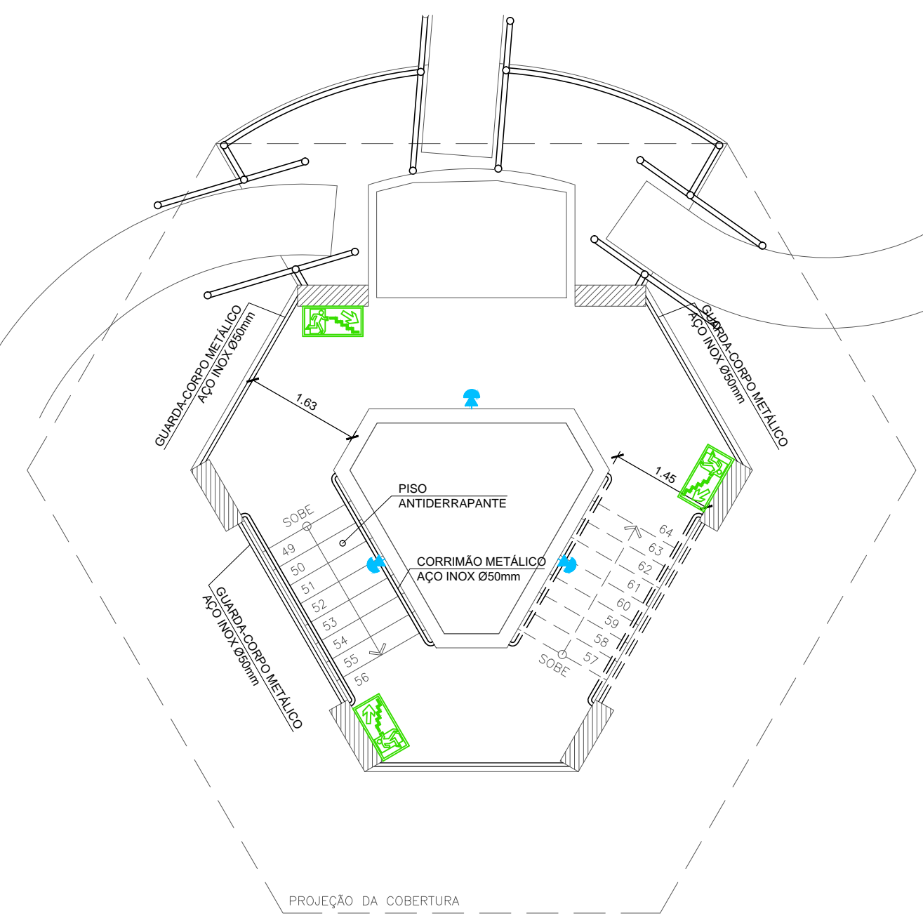
PLANTA BAIXA 2º PVTO - BLOCO 06 (TORRE) ESCALA: 1/75
