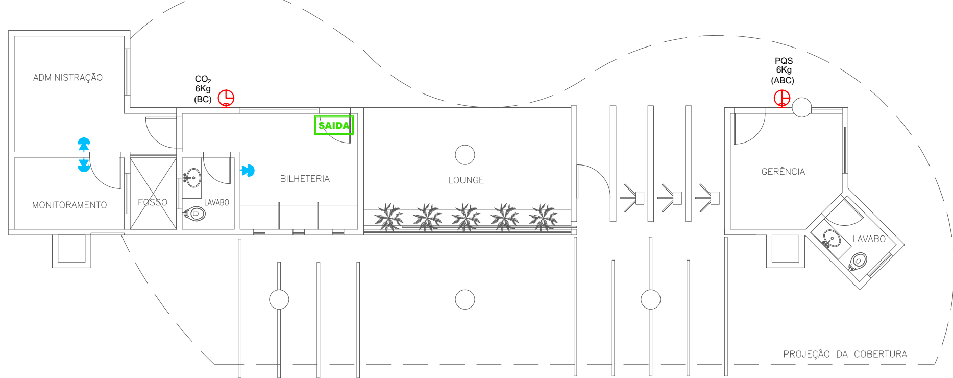
PLANTA BAIXA - BLOCO 15 (BILHETERIA/ADMINISTRAÇÃO) ESCALA: 1/75
