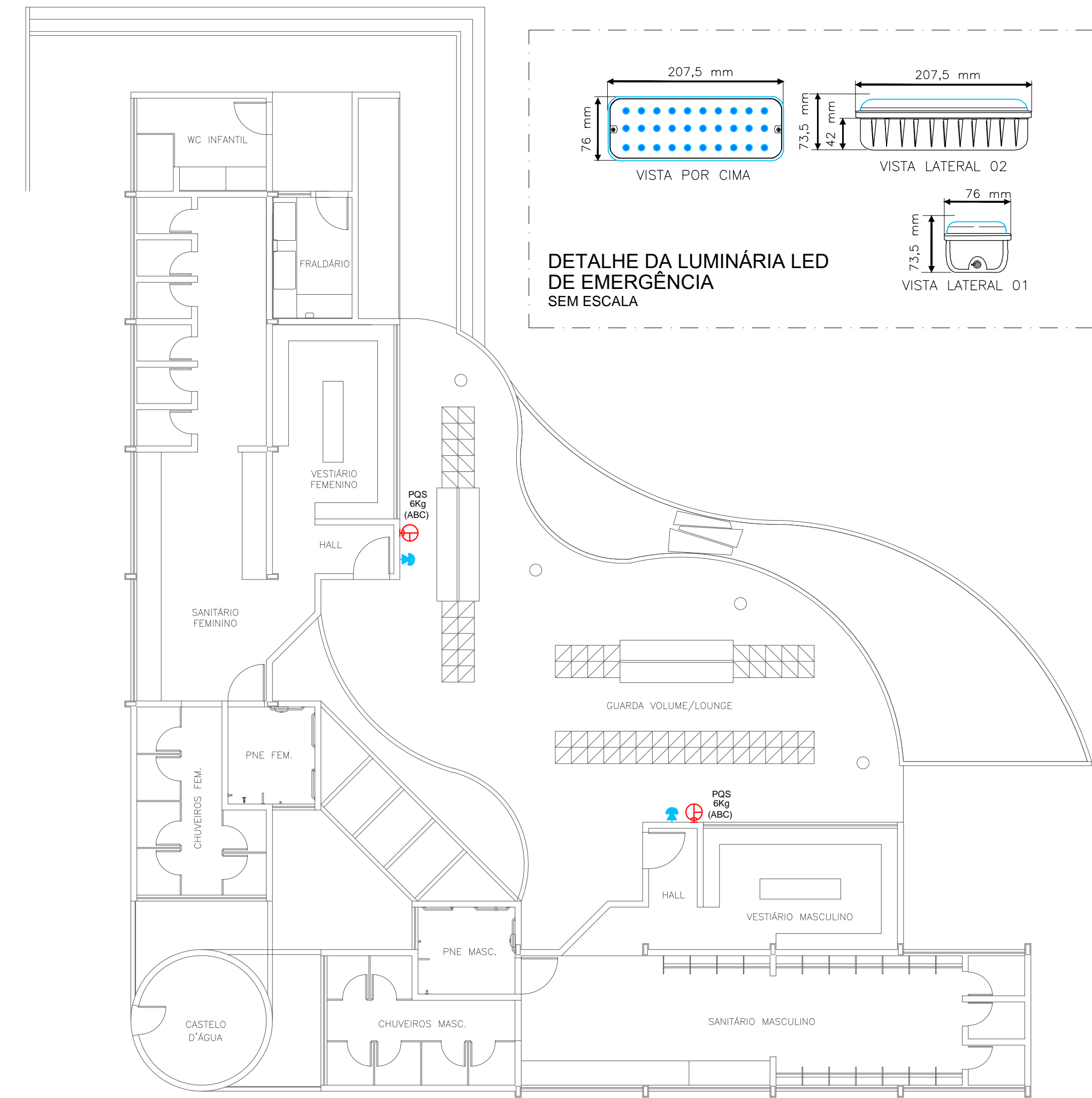
PLANTA BAIXA - BLOCO 01 (VESTIÁRIOS) ESCALA: 1/100
