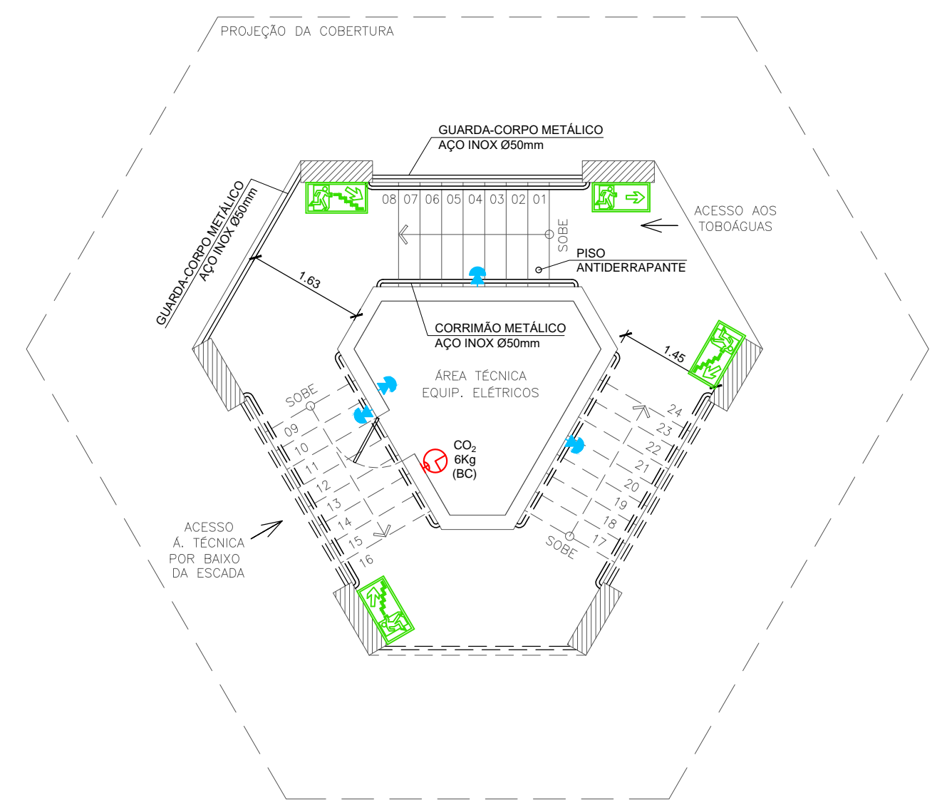
PLANTA BAIXA TÉRREO - BLOCO 06 (TORRE) ESCALA: 1/75
