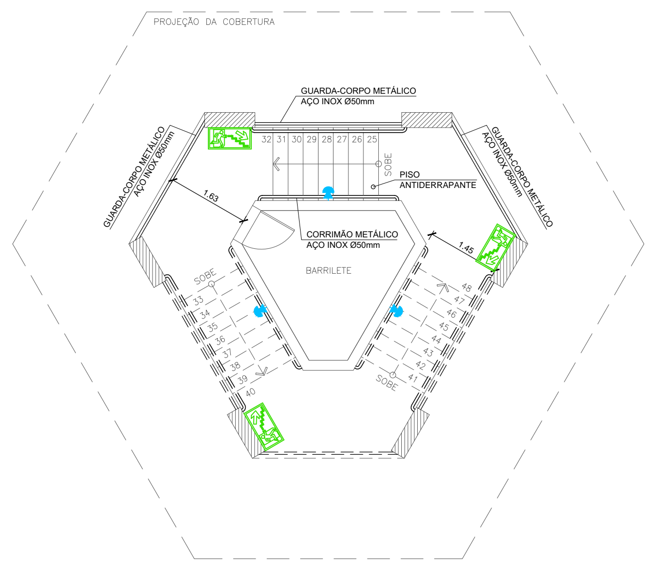
PLANTA BAIXA 1º PVTO - BLOCO 06 (TORRE) ESCALA: 1/75
